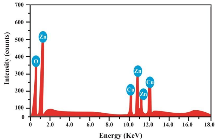
Fig.4. EDX spectrum of Cu doped ZnO
