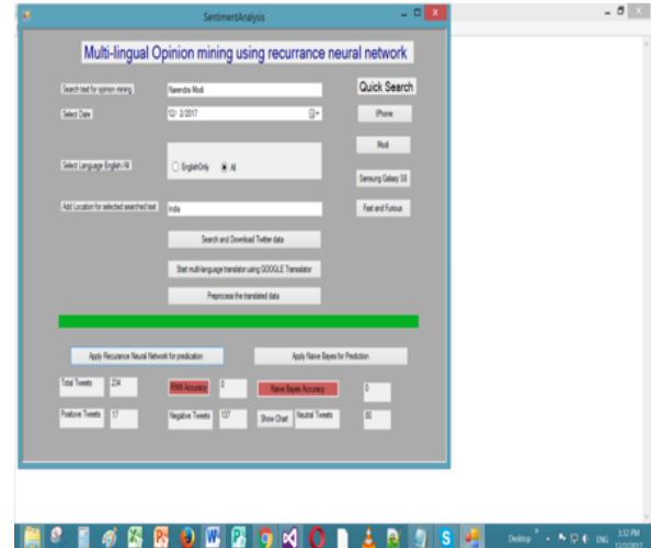
Fig. 10. Apply RNN
